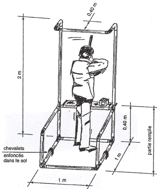
PLAN D'INSTALLATION.
