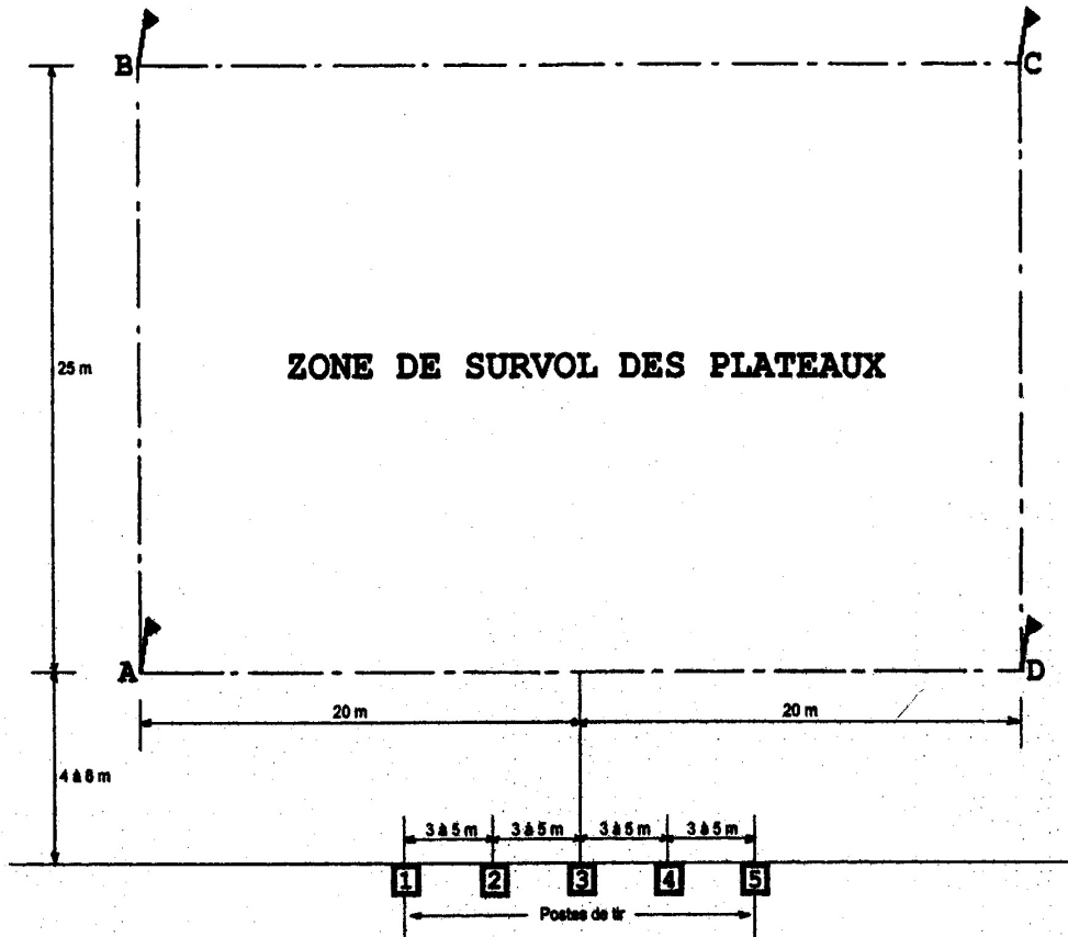
PLAN D'INSTALLATION.
